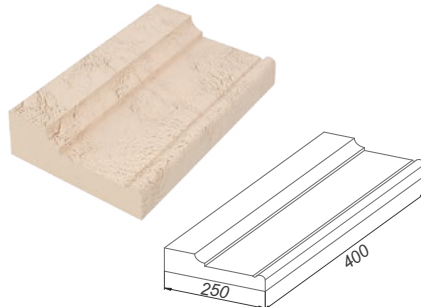
Наличник прямой АН6
