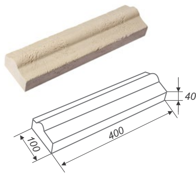
Карниз прямой АК1
