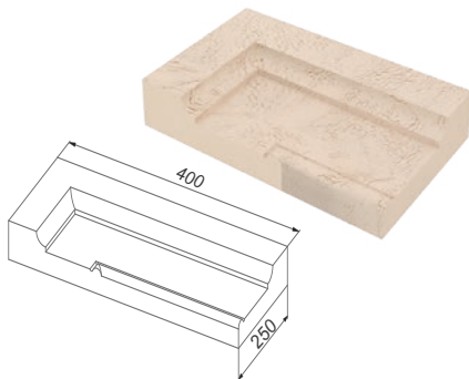
Наличник угловой левый АН6-Л
