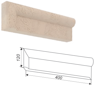
Наличник угловой левый АН5-Л
