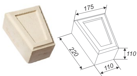
Замковый камень АЗ-4
