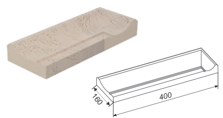
Наличник угловой правый АН3-П
