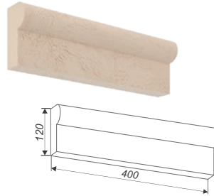
Наличник прямой АН5
