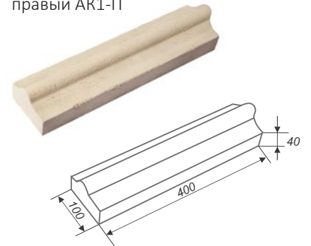
Карниз угловой правый АК1-П
