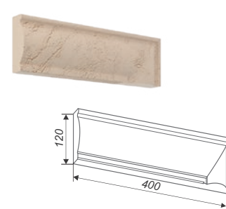
Наличник угловой правый АН3-П
