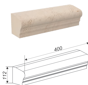
Карниз прямой АК4
