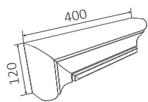
Оконный наличник прямой 004
