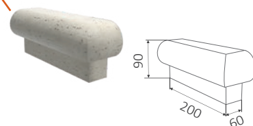
Рустовой камень обрезной 003
