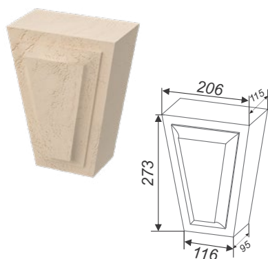
Рустовой камень поворотный АР1-ПОВ
