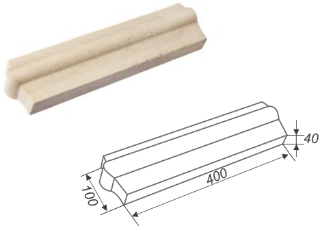
Карниз угловой левый АК1-Л
