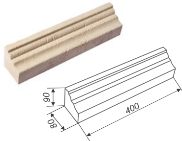
Наличник прямой АН1
