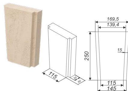
Замковый камень АЗ-3
