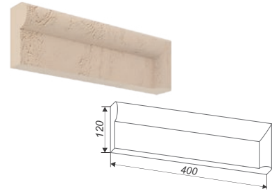
Наличник угловой правый АН5-П
