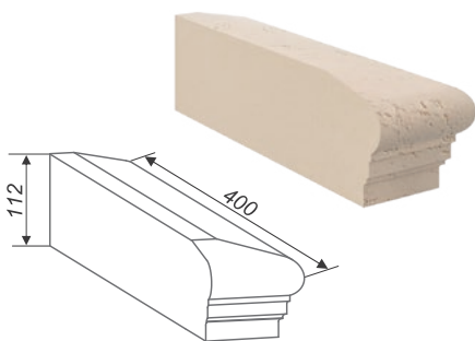
Карниз угловой левый АК4-Л
