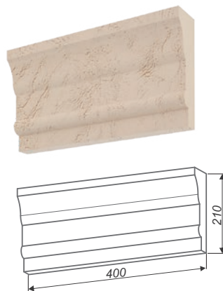
Карниз прямой АК3
