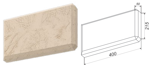
Рустовой камень поворотный АР2-ПОВ
