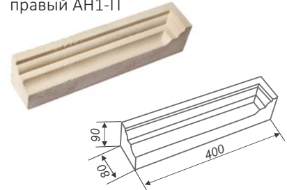
Наличник угловой правый АН1-П
