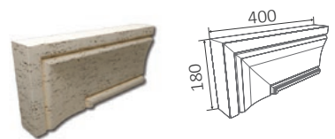
Дверной наличник угловой правый 005/1
