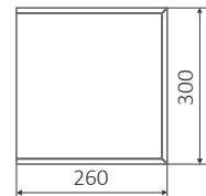
Рустовой камень обрезной 003
