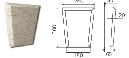
Дверной наличник угловой левый 005/2
