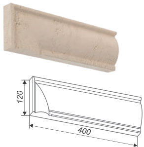
Наличник угловой левый АН3-Л
