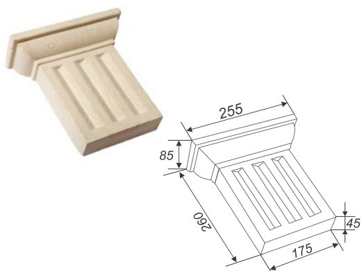
Рустовой камень обрезной АР1-ОБР
