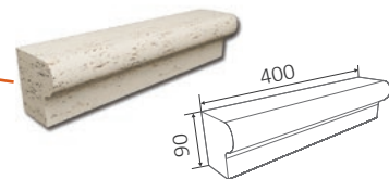
Подоконник угловой правый 006/1
