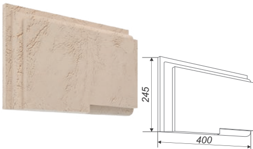
Наличник угловой левый АН6-Л
